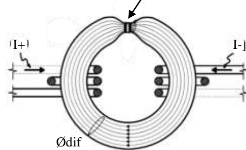
2.5: Detección del Flujo Magnético Diferencial.
