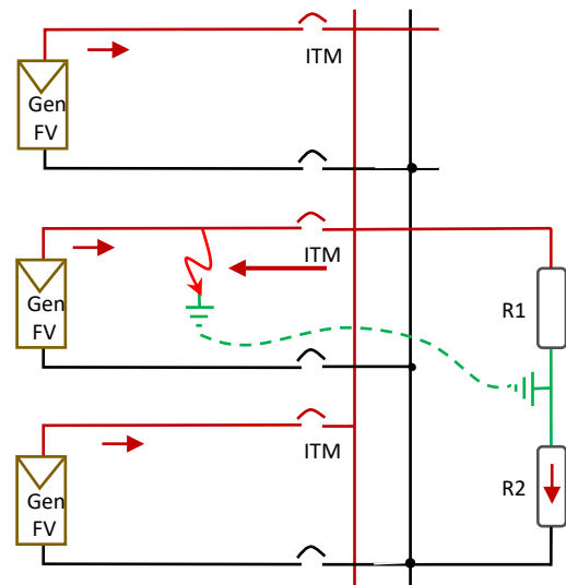
Figura 3.2. Trayectoria de Corriente de falla a tierra.
