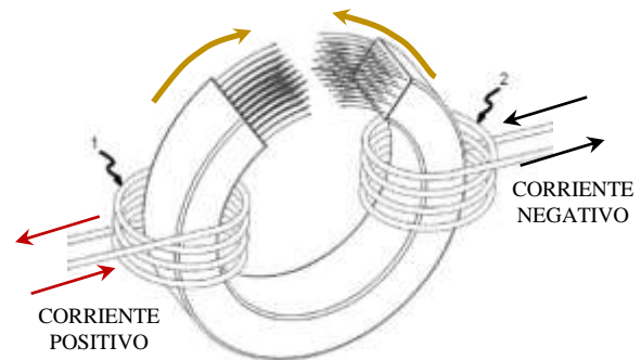
Figura 2.4: Núcleo Toroidal con arrollamientos y flujos magnéticos.
