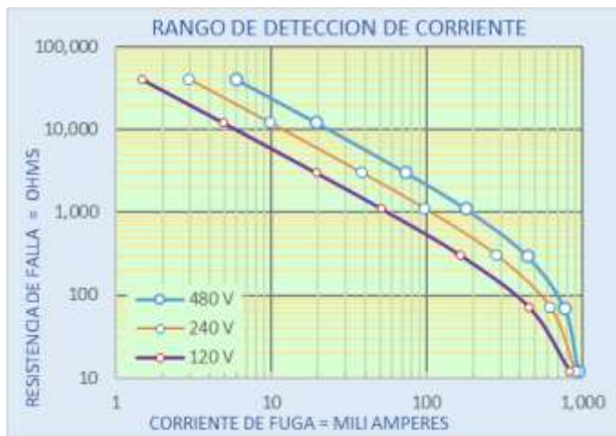
Figura 3.4. Corriente de falla en función de la resistencia de falla, para sistemas de 120, 240 y 480 Vcd.
