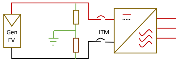
Figura 2.3: Sistema Aterrizado mediante un divisor de tensión.
