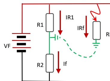
Figura 3.2. Trayectoria de Corriente de falla a tierra.
