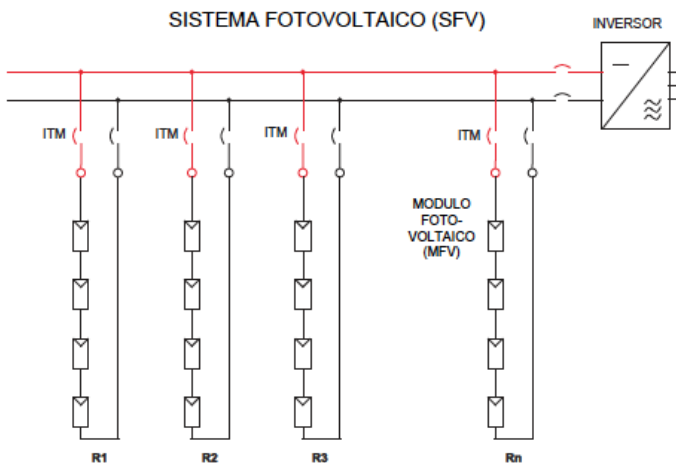
Figura 3.1 Ramas de Generadores Fotovoltaicos con protección por ITM.
