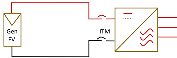
Figura 2.1: Sistema Flotante
