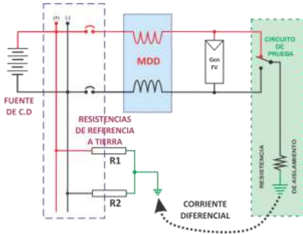
Figura 2.6: Principio de funcionamiento del detector de fallas a tierra.
