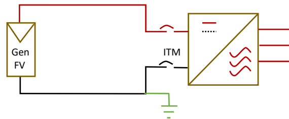
Figura 2.2: Sistema con Negativo Aterrizado.
