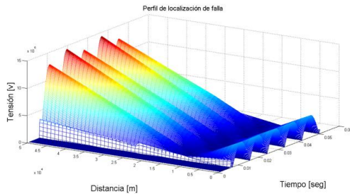
Fig. 7. Resultado gráfico de una falla a 10 km desde el nodo emisor.
