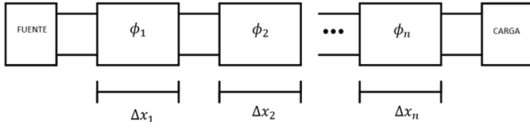
Fig. 4. Modelo de una línea de transmisión no uniforme.
