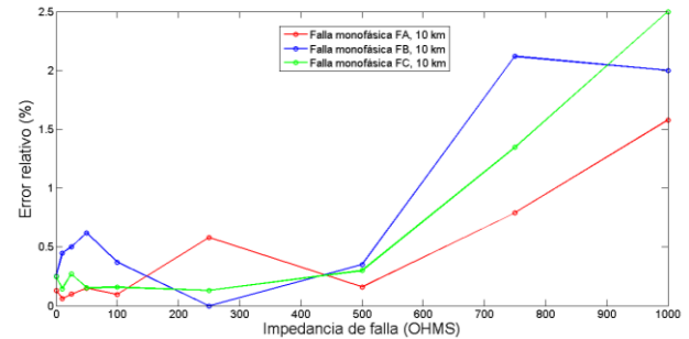
Fig. 10. Error relativo para la falla monofásica del caso 2.
