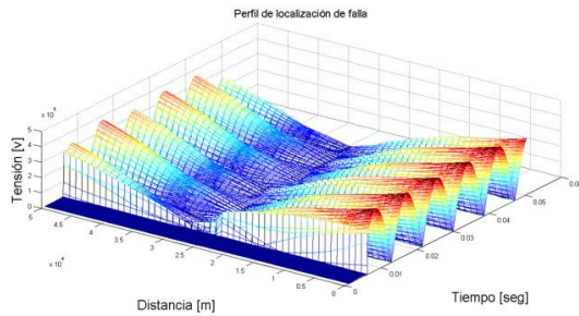
Fig. 8. Resultado gráfico de una falla a 25 km desde el nodo emisor.
