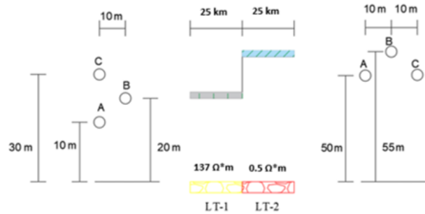
Fig. 5. Línea de transmisión no uniforme utilizada para probar el algoritmo de localización de fallas.
