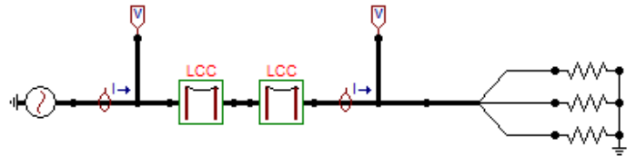
Fig. 6. Modelo en ATPDraw utilizado para obtener las muestras de tensión y corriente en los extremos de la línea.
