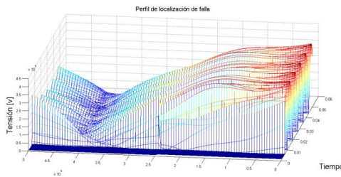
Fig. 9. Resultado gráfico de una falla a 40 km desde el nodo emisor.
