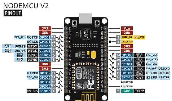
Fig. 3. Diagrama de pines del SoC NodeMCU.
