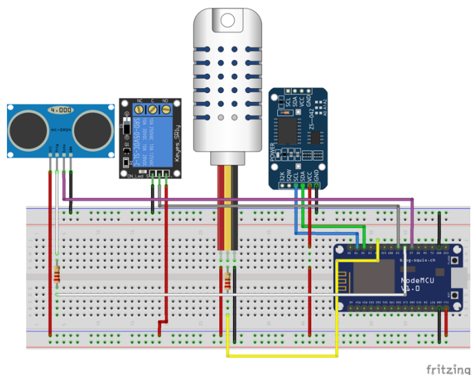
Fig. 8. Diagrama de conexión de sistema de control, apartado electrónico.
